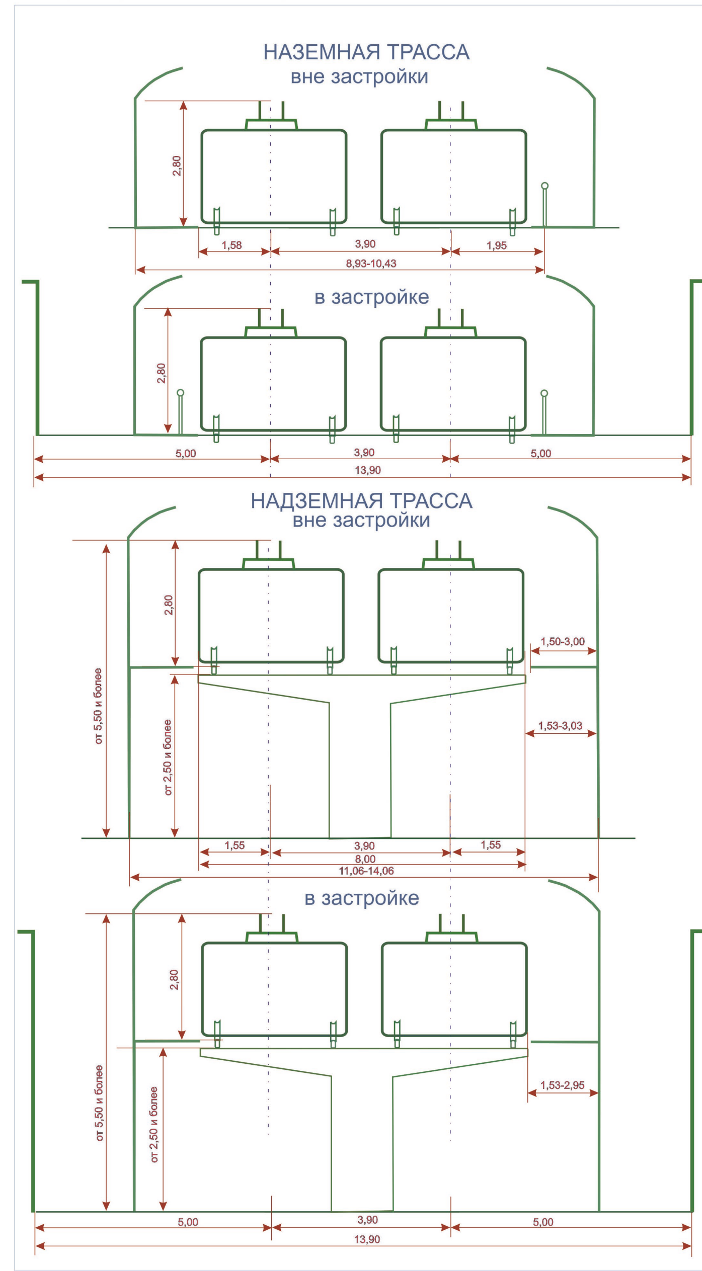
Коридоры станций двухколейной линии СТЮ на перегоне
