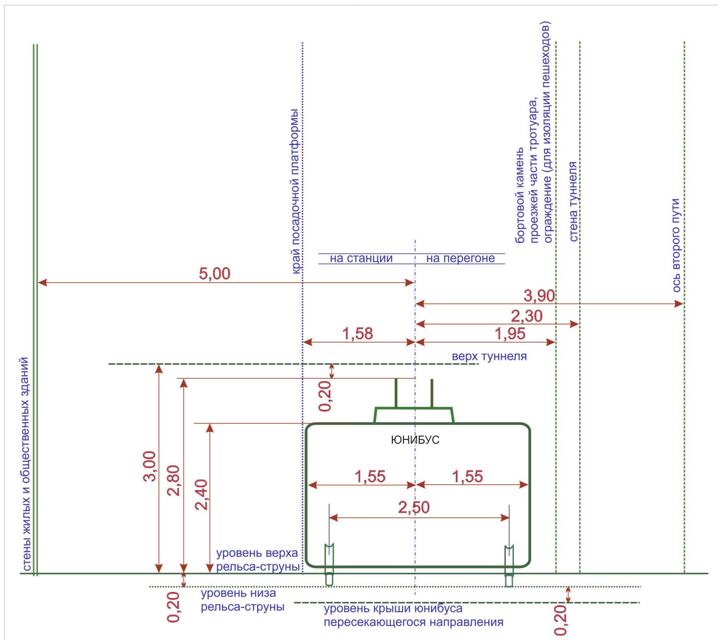
Габариты линии СТЮ на пересечениях
