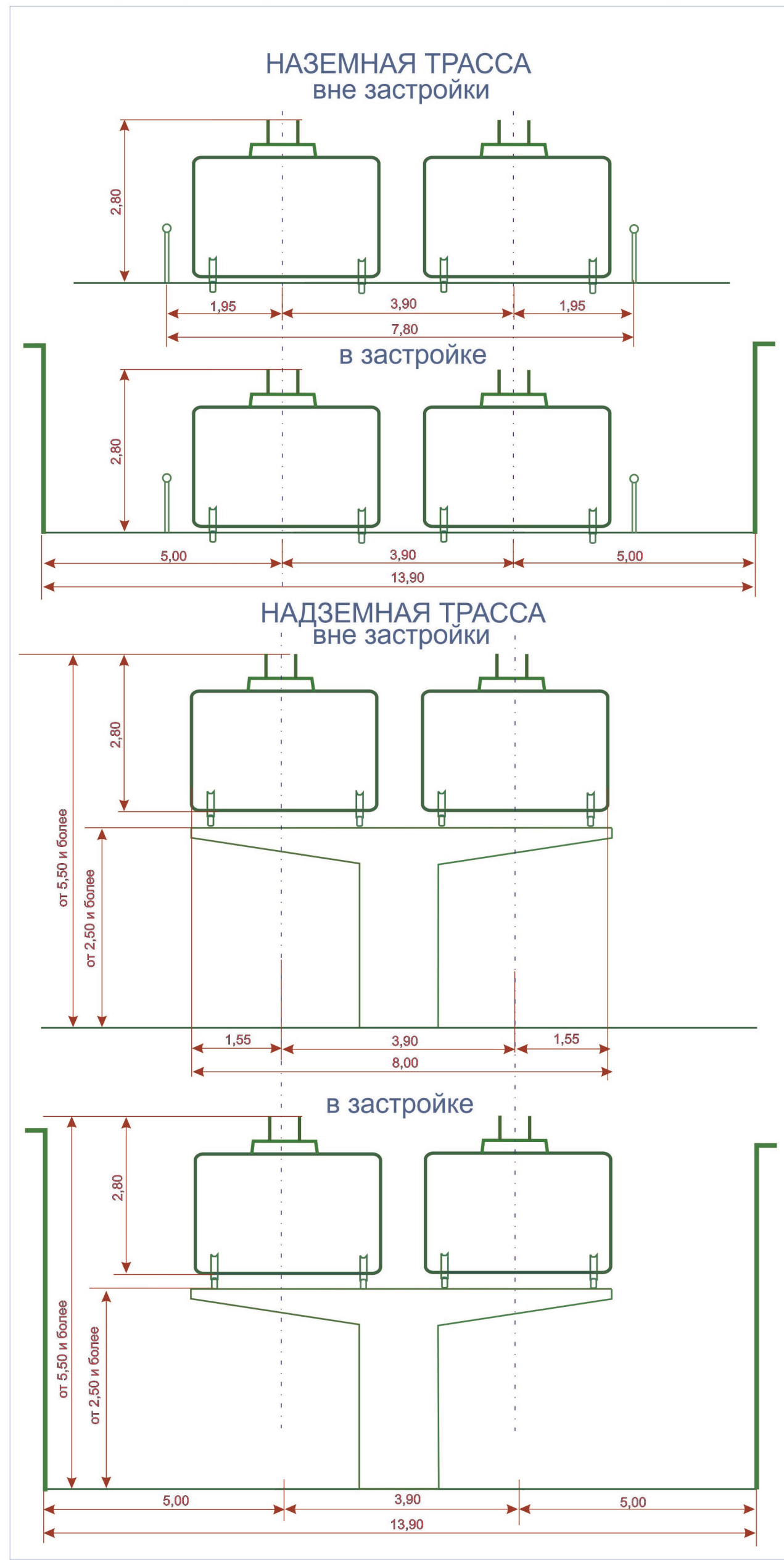
Коридоры двухколейной линии СТЮ на перегоне
