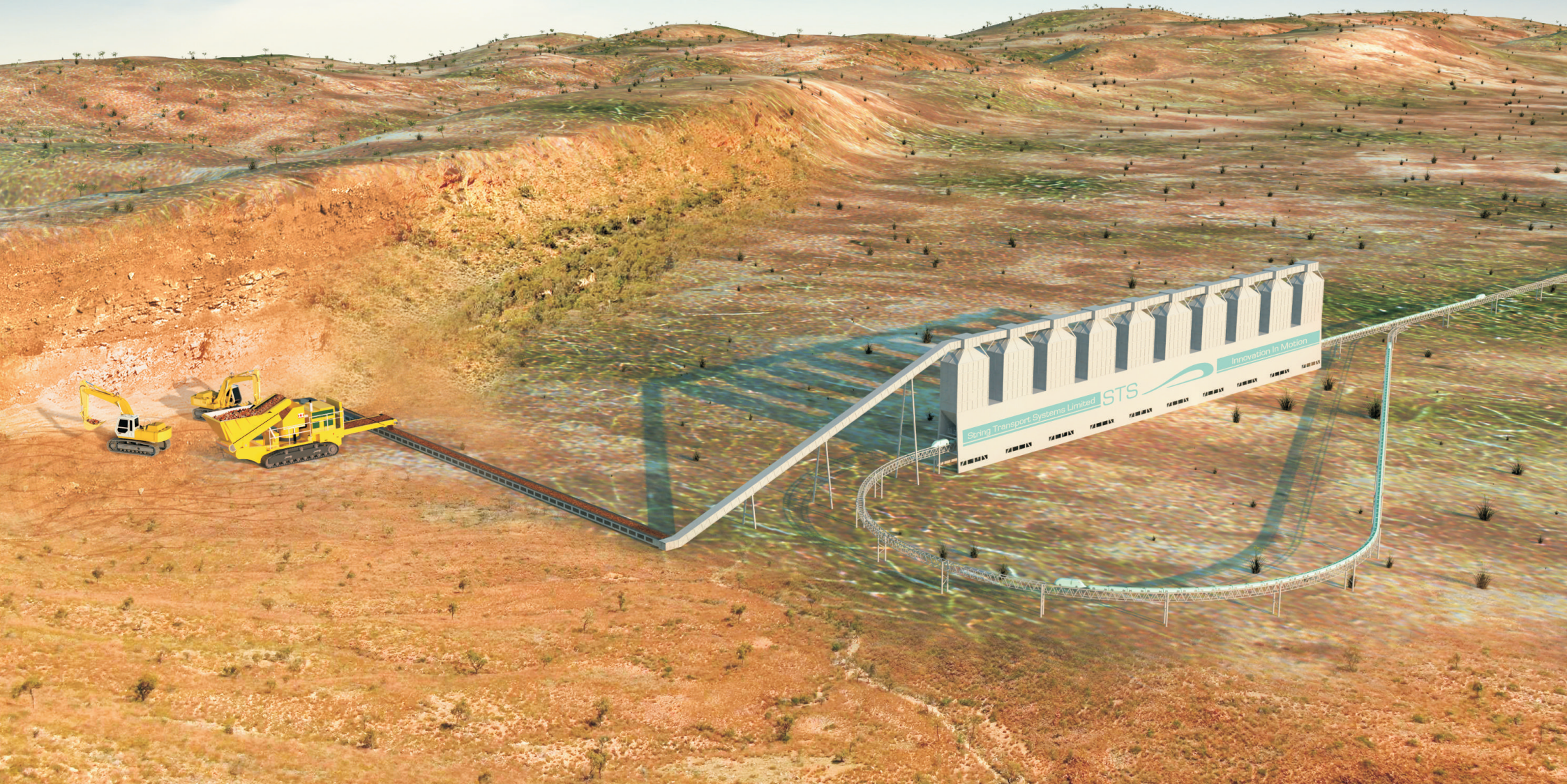
Добыча руды и её погрузка в СТЮ
