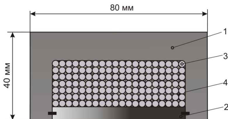
Рис. 2. Конструкция подвешенного струнного рельса в масштабе 1:1 в виде предварительно напряжённой на анкерные опоры провисающей ванта с верхней и боковыми ездовыми поверхностями (пролёты до 1000 м; скорость движения рельсового автомобиля в середине пролёта — до 120 км/час):
