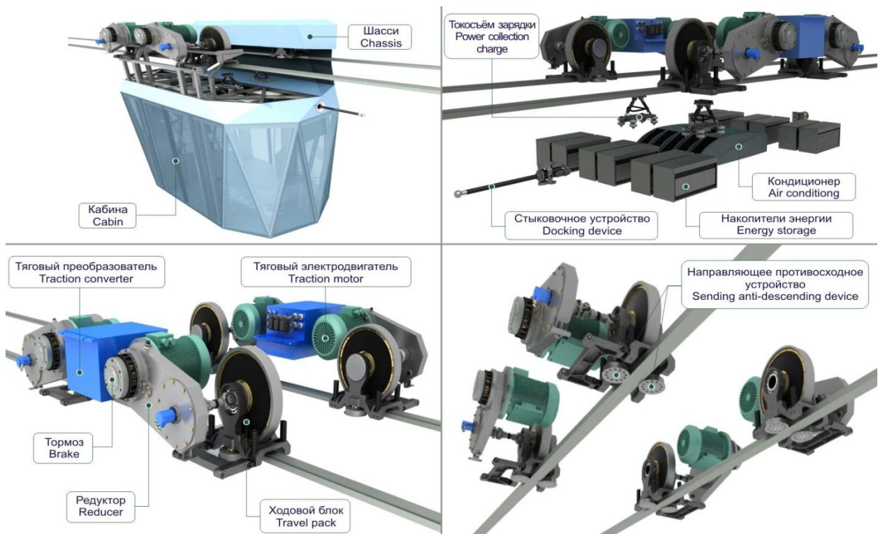
Рис. 3. Конструкция городского подвешного пассажирского юнибуса вместимостью 30 пассажиров (скорость движения — до 150 км/ч)
