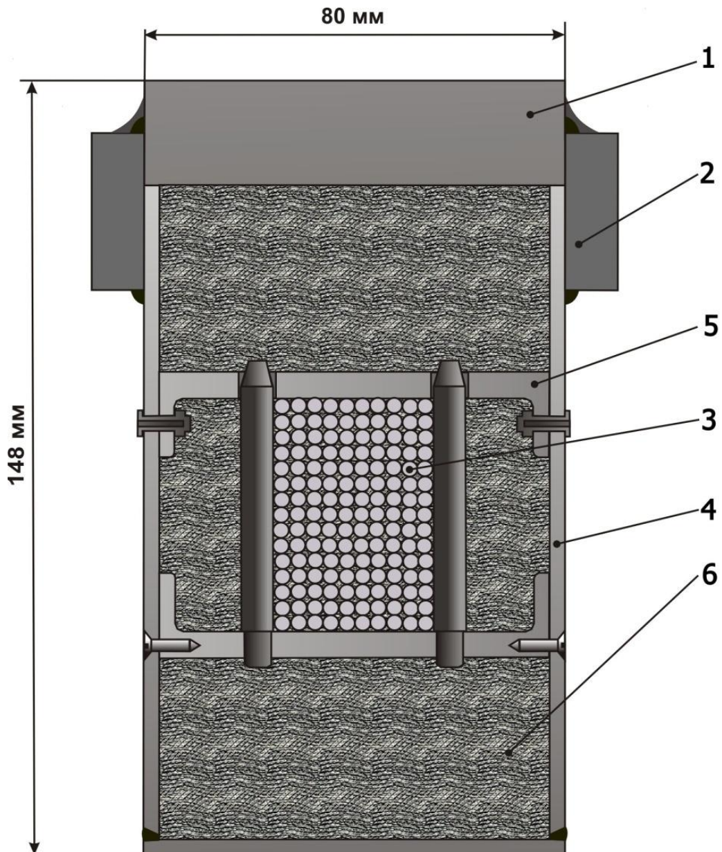
Рис. 1. Конструкция городского навесного струнного рельса в масштабе 1:1 в виде предварительно напряжённой на анкерные опоры сталежелезобетонной балки с верхней и боковыми ездовыми поверхностями (для пролётов 40 м; скорость движения рельсового автомобиля — до 120 км/ч):
